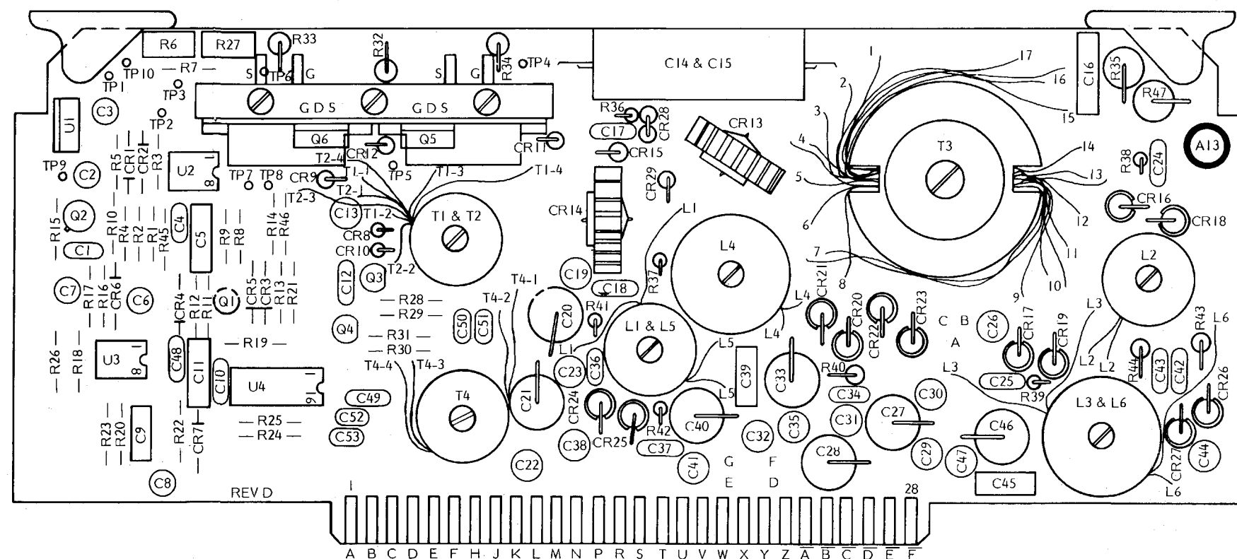
A13 PCB
